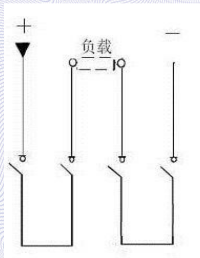
4P 外形接线图(DC1000V)
