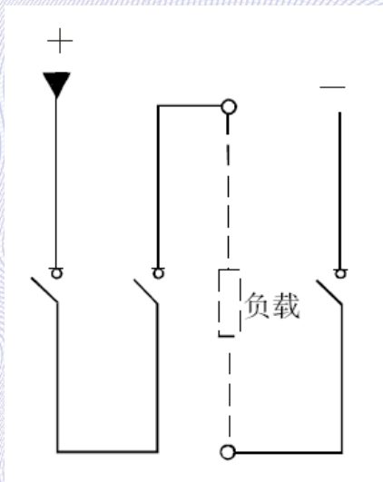
3P 外形接线图(DC500V)
